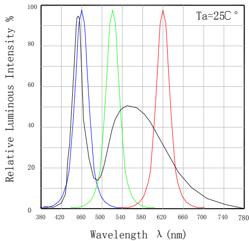
光谱特性图
