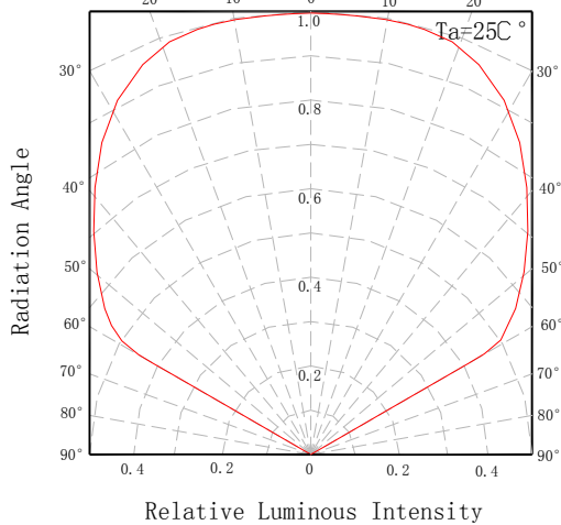
发光角度图
