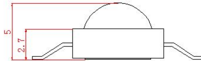
侧视图
