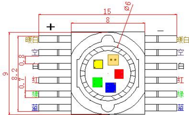
俯视图
