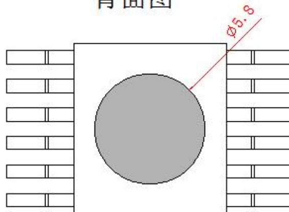
背面图
