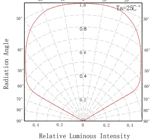
发光角度图
