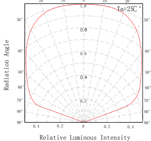
发光角度图
